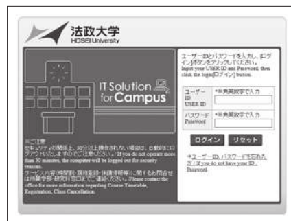
PC版画面
