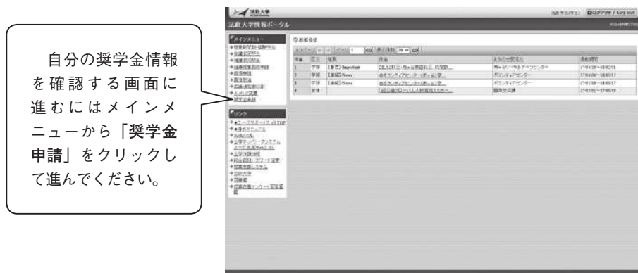
PC版画面
