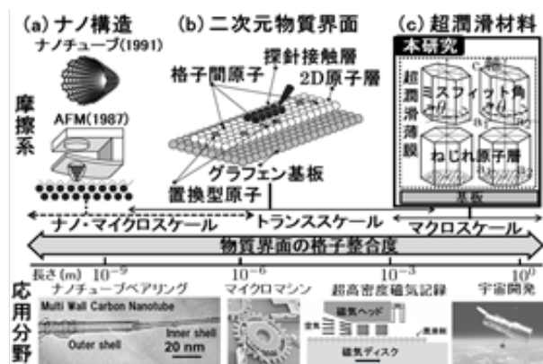
図1 ナノ-マクロスケールに見られる摩擦。摩擦がスケール間で異なるとき遷移(トランス)領域が現れる。
