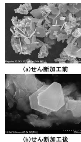
図5 WS 2 原子層のせん断変形
